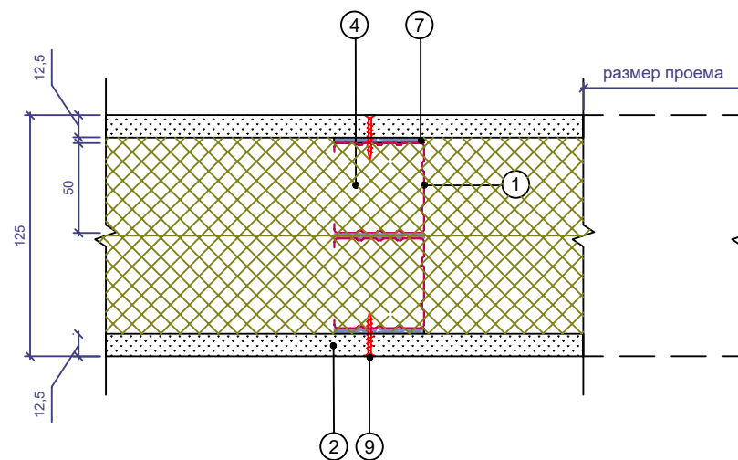
Обычный проем
