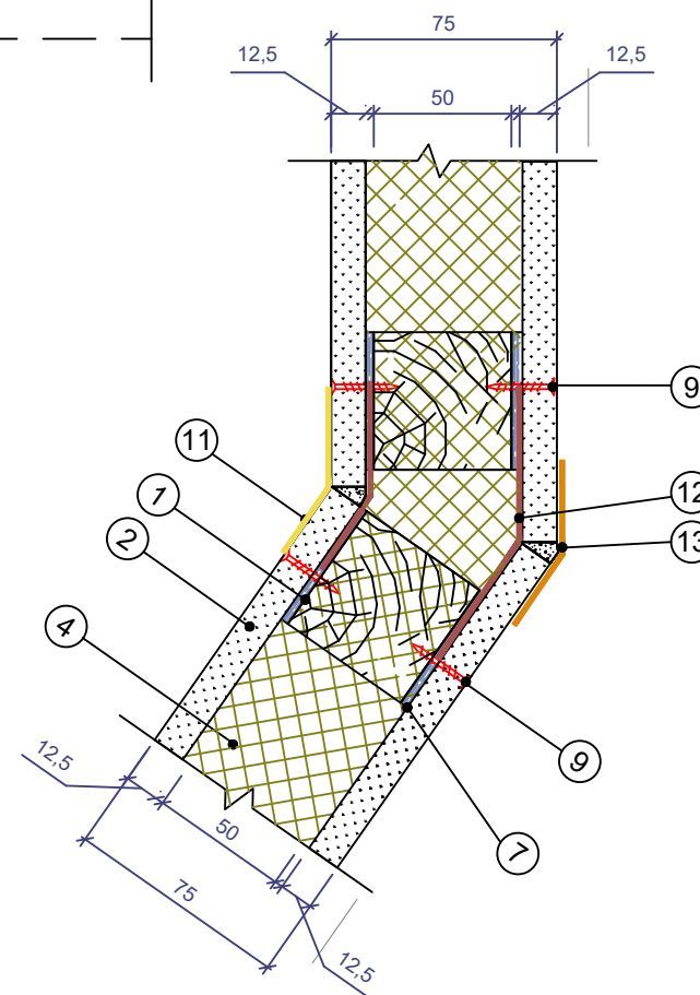
Стык перегородок под углом не равным 90°
