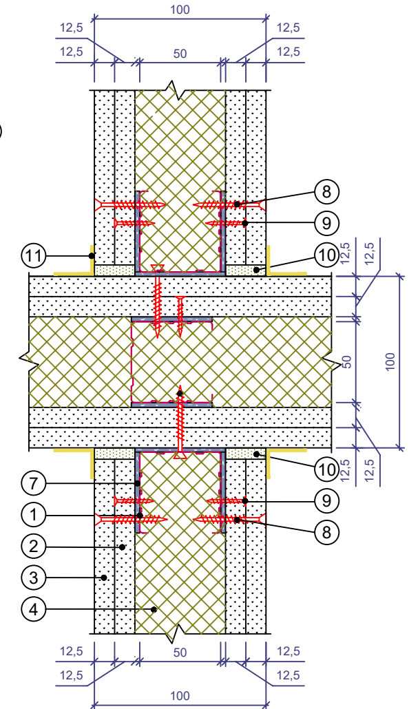
Стык перегородок
