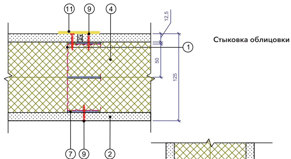
Стык перегородок
