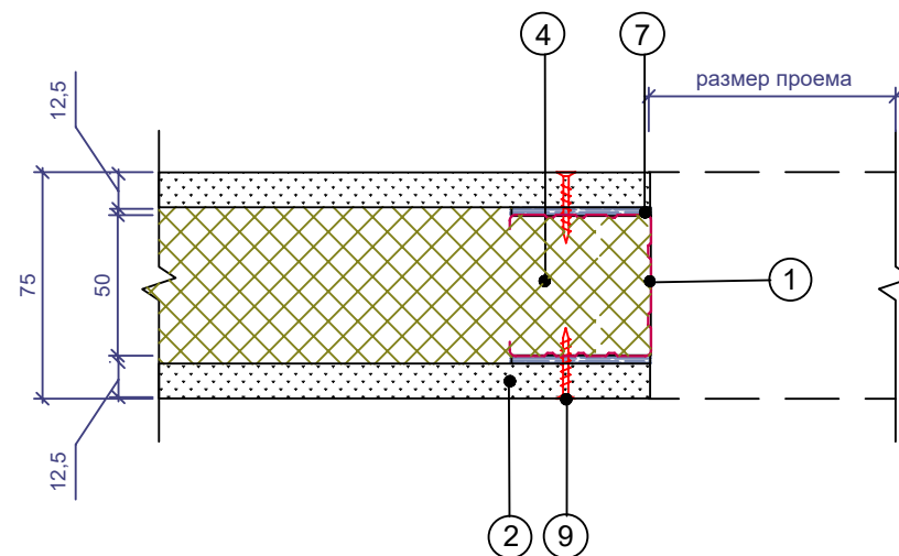
Стык перегородок
