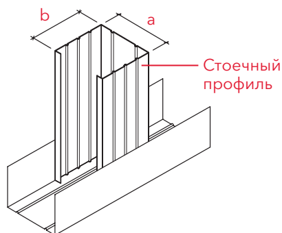
Геометрические размеры стоечных профилей
