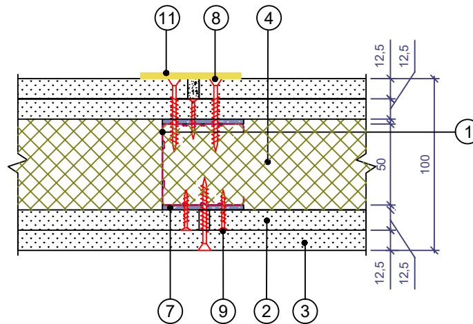
Стыковка облицовки
