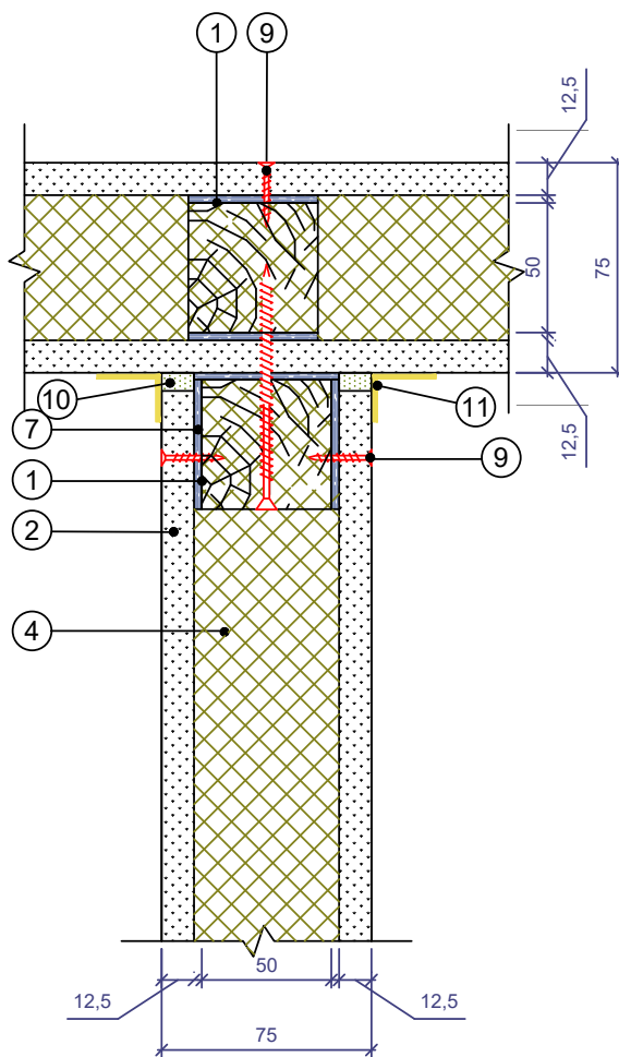
Примыкание перегородок под углом 90°
