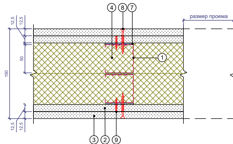
Обычный проем
