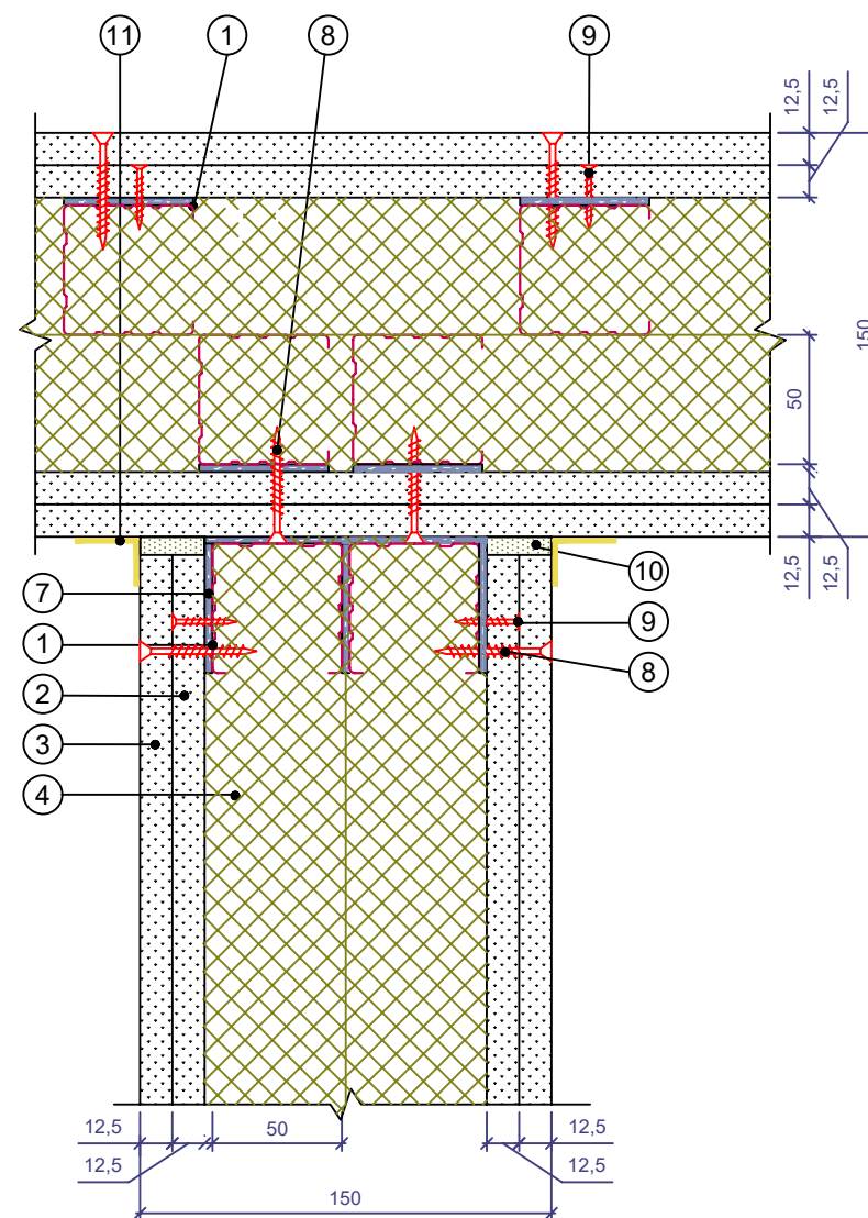
Примыкание перегородок под углом 90°
