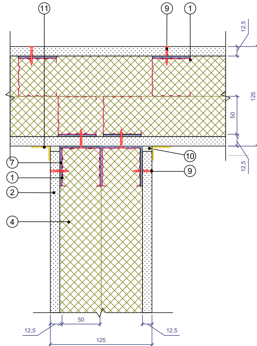
Примыкание перегородок под углом 90°
