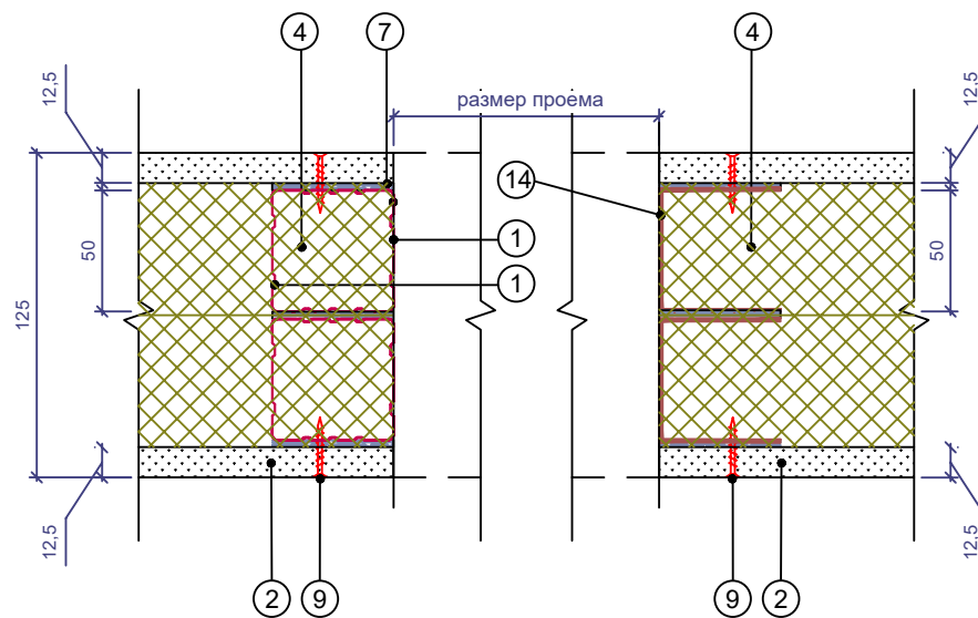
Обычный проем
