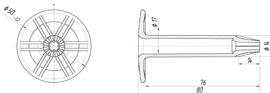
Схема телескопического крепежа 80 мм
